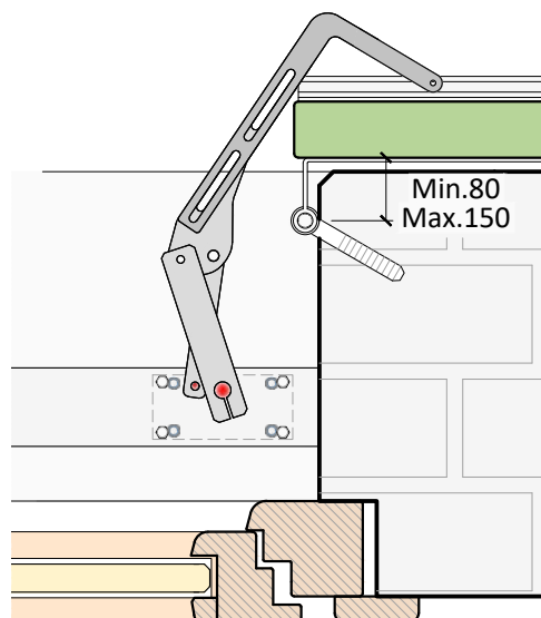
Bandella zancata
