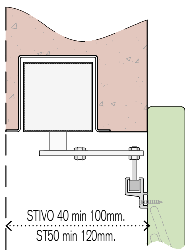
Autom. incassata
