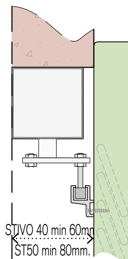
Binario sottostante
