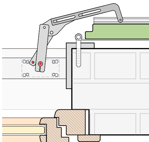
bandella dritta
